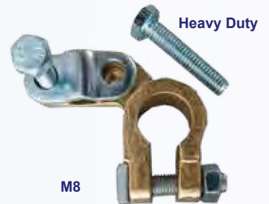
M8 AP.208 - 10 Kabel / cable / câble Ø 25 - 70 mm 2
